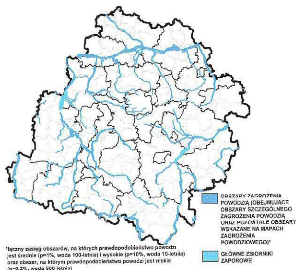
Rys. 33. Zagrożenie powodziowe
