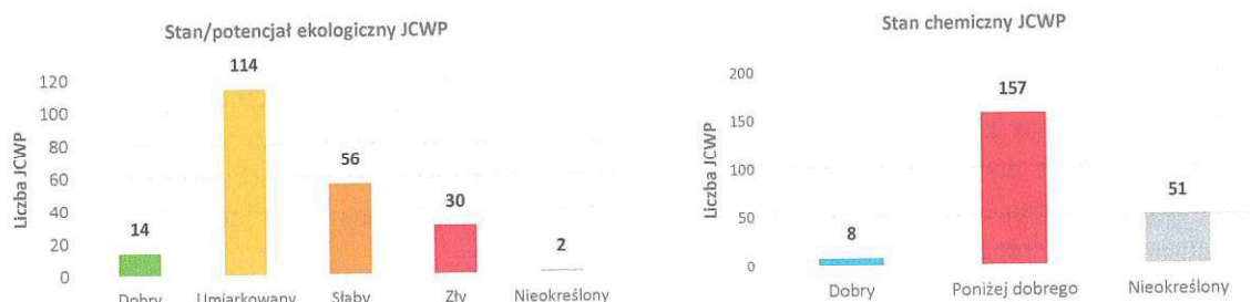
Rys. 29. Stan ekologiczny i chemiczny JCWP w latach 2014-2021
