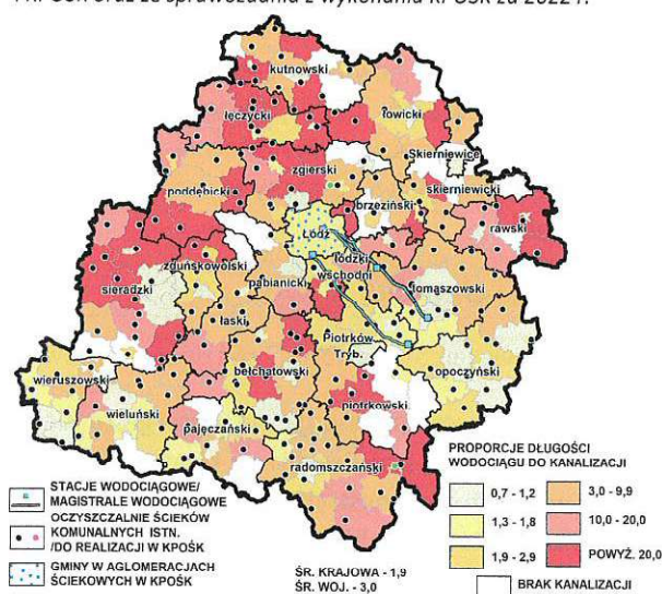
Rys. 58. Gospodarka wodno-ściekowa w woj. łódzkim w 2023 r. Źródło: Opracowanie własne na podstawie danych BPRWŁ, GUS i KPOŚK oraz ze sprawozdania z wykonania KPOŚK za 2022 r.
