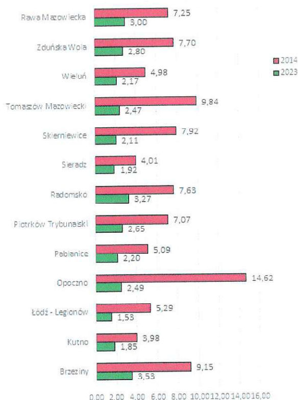
Rys. 35. Ponadnormatywne wartości średnioroczne poziomu stężenia benzo(a)pirenu w pyłach PM10 w województwie łódzkim odnotowane w wybranych stacjach pomiarowych w latach 2014 i 2023 r. [ng/m³]
